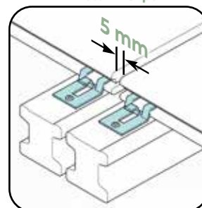
Doppelte Unterkonstruktionen aus Verbundholz + Distanz-Clips
