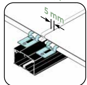
Unterkonstruktion aus Silvadec®-Aluminium + Distanz-Clips
