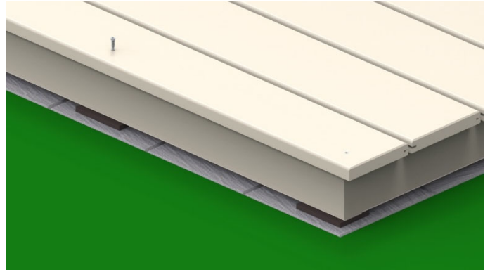
Bild 34. Schieben Sie die abgeschnittene Terrassendiele mit der Nutseite auf die RASK-Clipse. Anschließend wird die Diele mit einer Terrassenschraube min. 5 x 60 V2A alle 50 cm auf der Unterkonstruktion verschraubt. Die Schrauben sollten gleichmäßig max. 1 mm tief versenkt werden.
