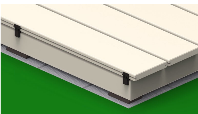
Bild 37. Wenn alle Oberteile eingesteckt sind, muss die Terrassendiele runtergedrückt werden und dadurch wird das Oberteil vom Startclip arretiert.
