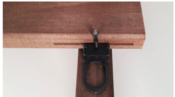
Bild 42. Der RASK-Clip muss mittig in der Ausfräsung positioniert werden.
