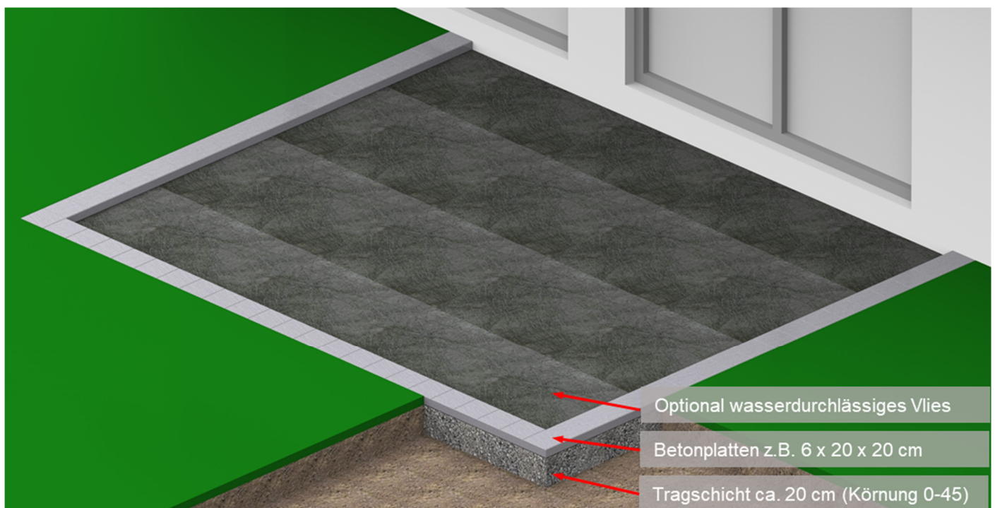
Bild 5. Bei der Verwendung von Verstellfüßen statt Betonplatten, kann auf die Bettungsschnitt verzichtet werden. Bei Verwendung eines dunklen bzw. schwarzen Unkrautvlieses fallen die Verstellfüße in den Fugen nicht mehr so auf. Das Unkrautvlies muss wasserdurchlässig sein und sollte ca. 10 cm überlappen.
