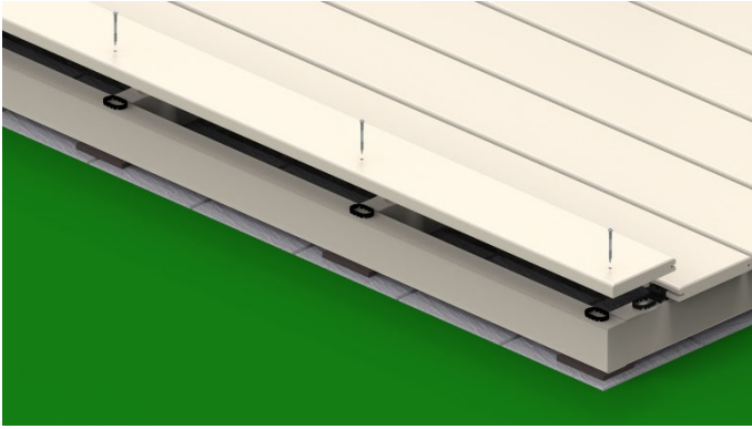
Bild 33. Schneiden Sie bei der letzten Terrassendiele immer auf einer Seite die Nut ab. Wenn die Diele nicht auf die erforderlich Breite geschnitten wird, kann die obere Nutwanne während der Nutzung leicht abbrechen.
