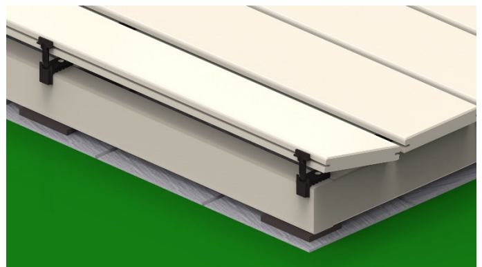
Bild 36. Die Diele wird danach schräg auf den RASK-Clip geschoben und anschließend können die Oberteile in die Nut der Diele gesteckt werden.
