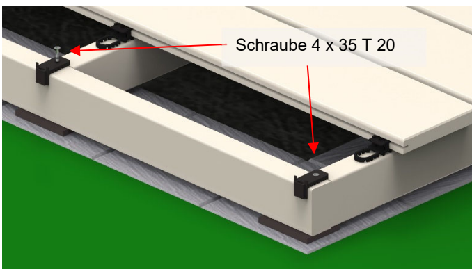
Bild 35. Zuerst wird nur das Unterteil vom Startclip mit den Schrauben 4 x 35 mm (T 20) auf die vordere Holzunterkonstruktion geschraubt.
