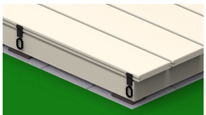
Bild 38. Da die vordere genutete Kante der Terrassendiele sehr bruchempfindlich ist, muss immer eine Blende montiert werden. Für die Montage der Blende verwenden Sie wieder Teilstücke vom RASKCLIP. Diese Teilstücke stellen den richtigen Abstand sicher.
