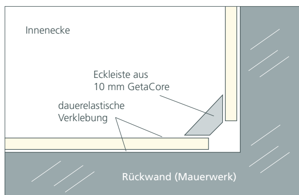
Beispiele einer Eckverbindung (Quelle: GKV. Technisches Merkblatt 92, Seite 22, Stand November 2004)
